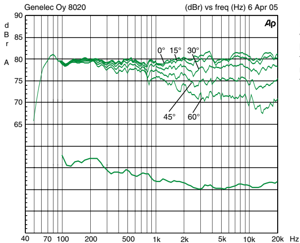
Kuva 5: Ylemmät käyrät esittävät 8020C:n taajuusvasteen eri kulmista mitattuna (kaiutin pysyasennossa, mittauasetäisyys 1 m). Alempi käyrä on kaiuttimen tehovaste.
